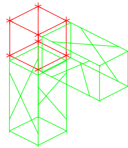
Dado 90 Deg Corner (2)
